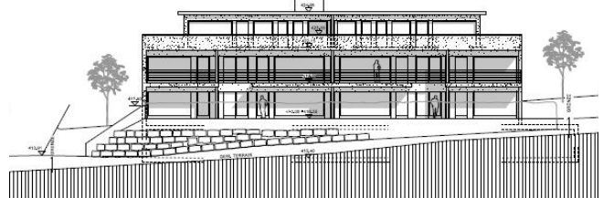
Südfassade
