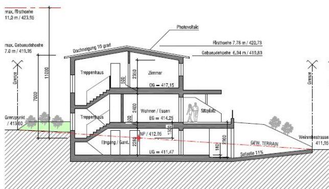
Querschnitt 1-1
