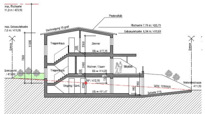
Querschnitt 1-1
